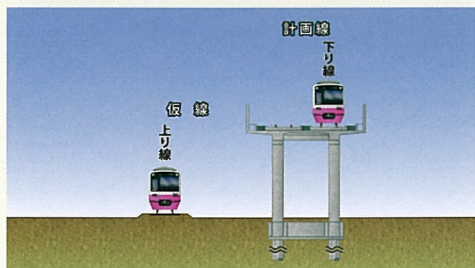
④ 計画下り線切替・仮下り線撤去
