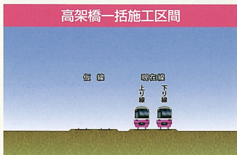
① 2線分の仮線用地を確保し仮線を敷設
