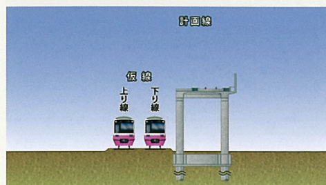
③ 上下線が仮運行中
