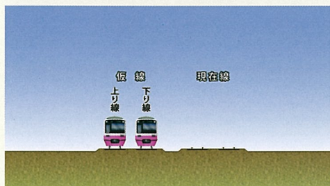
② 現在上下線を仮線に切替
